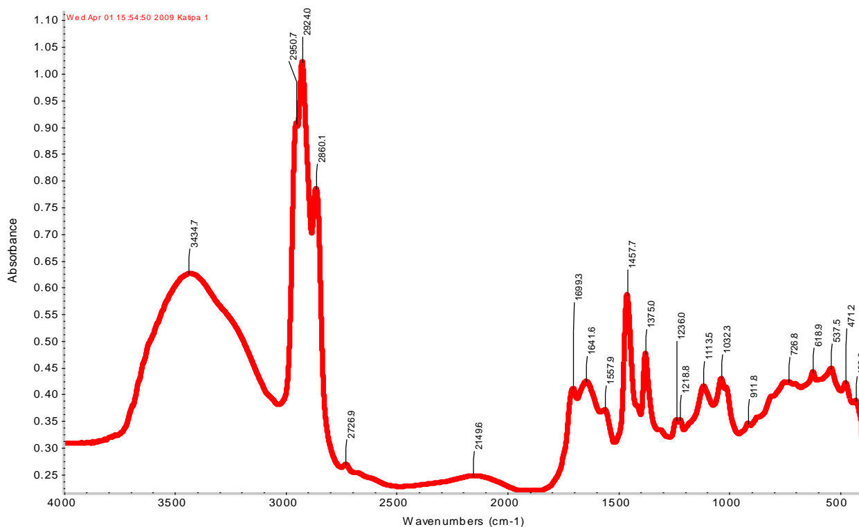
Рис. 2. ИК-спектры образца K-1
