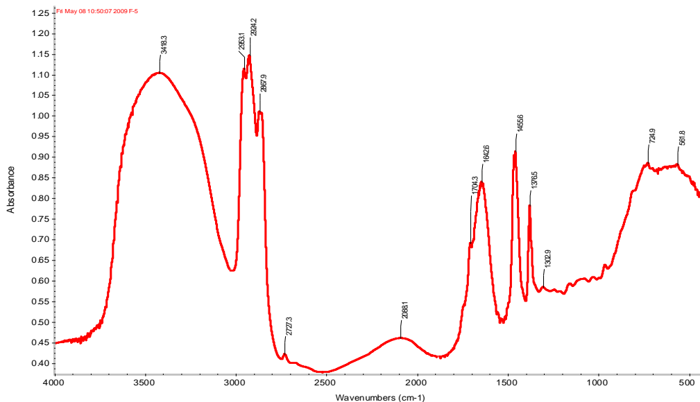
Рис. 1. ИК-спектры образца F-1
